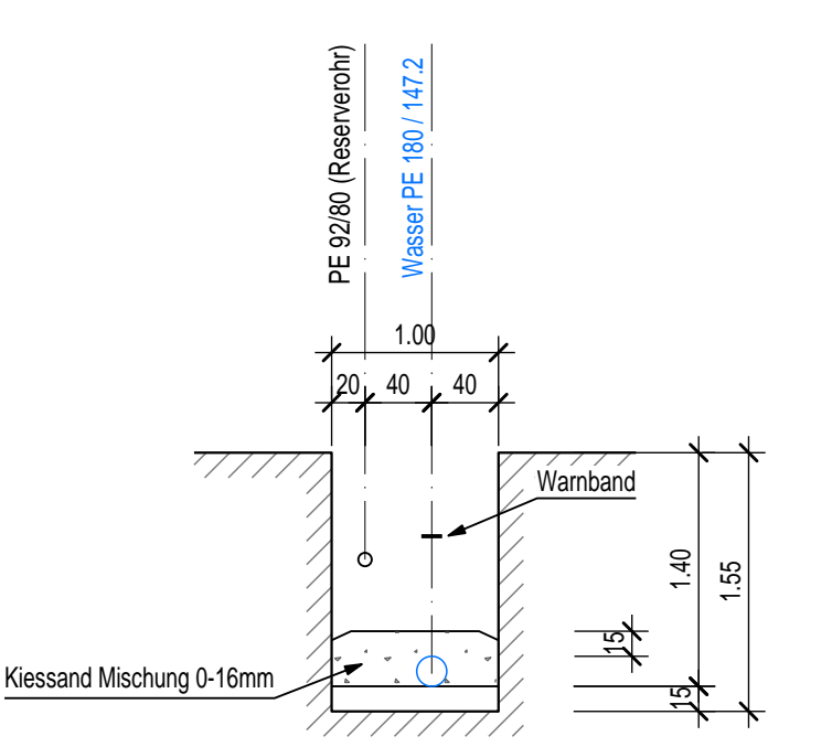
Grabenprofil 1:50
